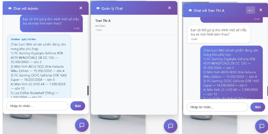
Hình 3.48. Chatbox
