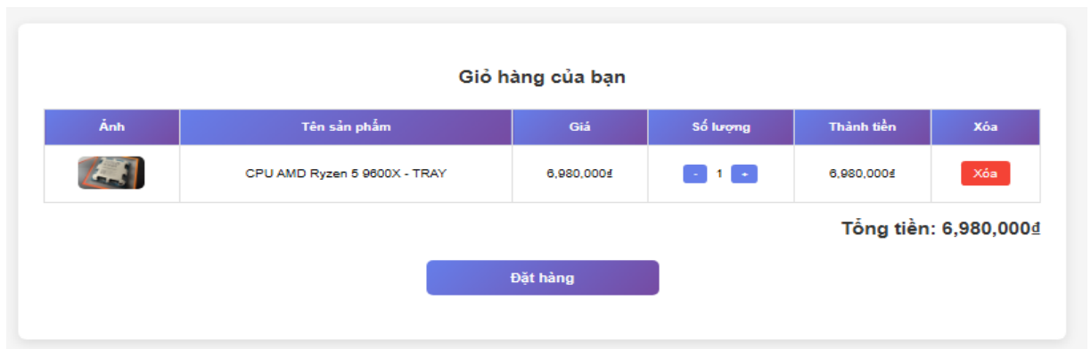
Hình 3.33. Giỏ hàng
